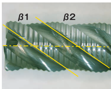
外周刃の不等リード
