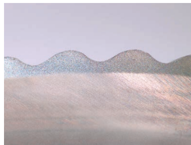
外周刃のラフィング形状
