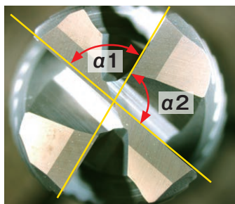
底刃の不等分割
